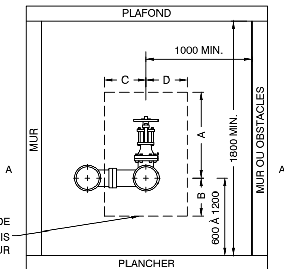
COUPE A-A' AUCUNE ÉCHELLE
